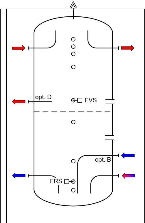
Bild 4: HT-Systempufferspeicher
